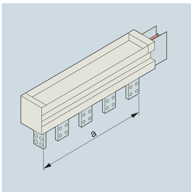
侧出线
