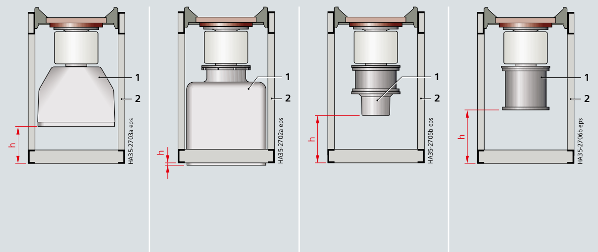
8DA10, 8DB10 和 8DA11/12 柜体连接的电缆头和母排
