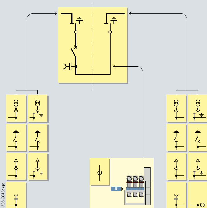
母线分段柜 (2 面柜体)
