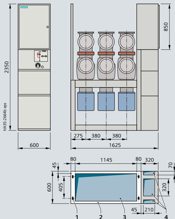
PT柜
