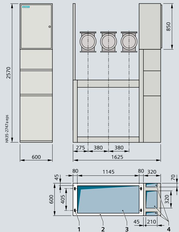
辅柜
