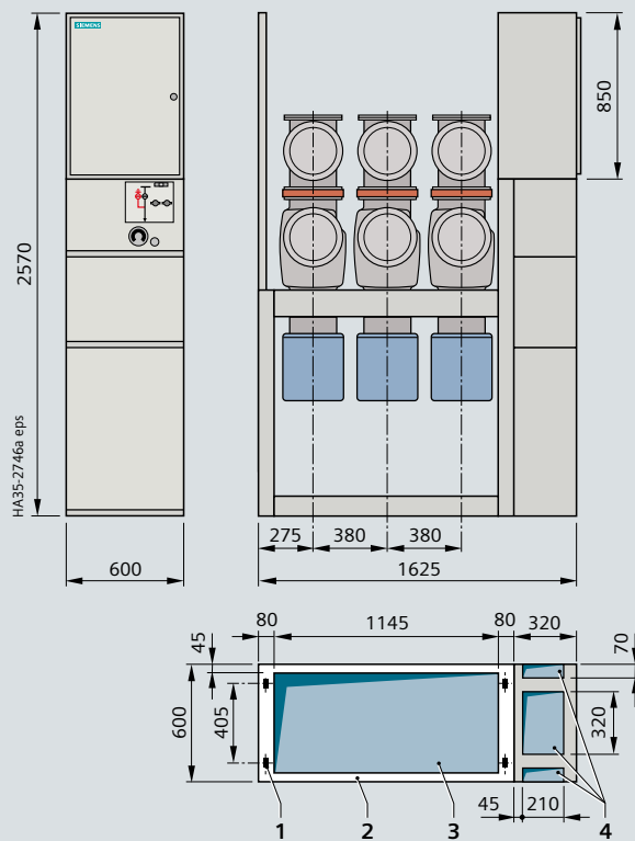
PT 柜
