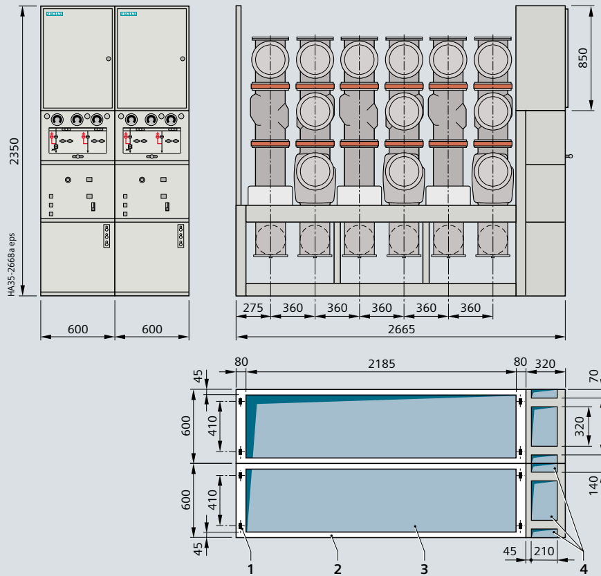
母线分段柜，最大电流 2500 A (母线系统 1 和 2)
