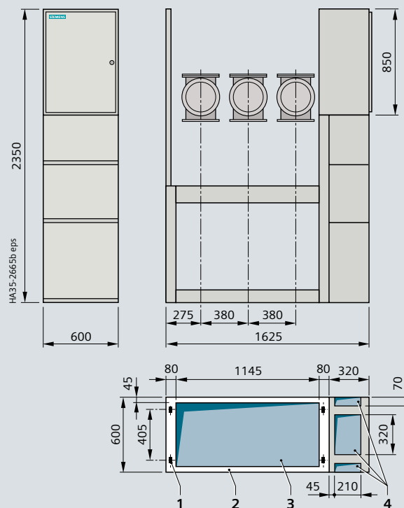
辅柜
