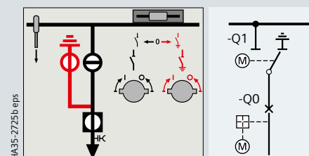
馈线接地
