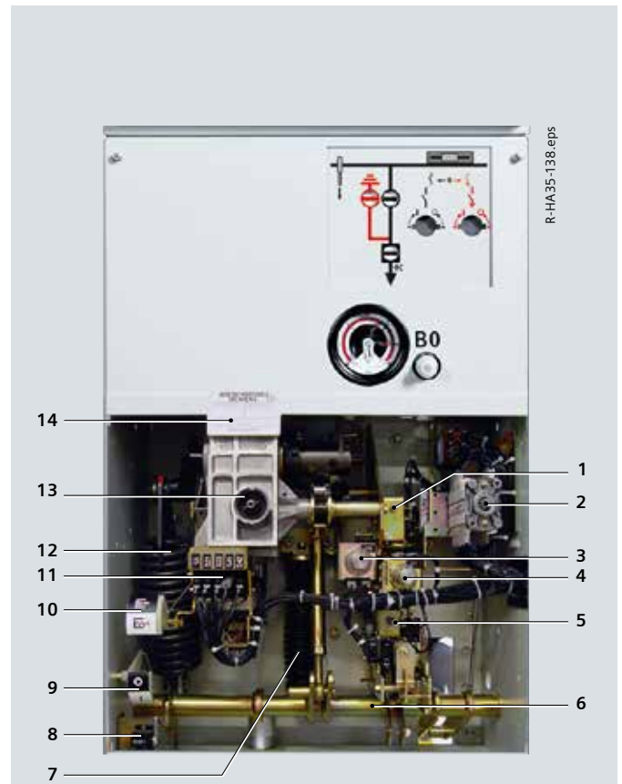
8DA 和 8DB 真空断路器操作机构 3AH49
