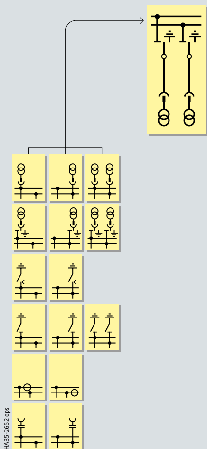
PT 柜
