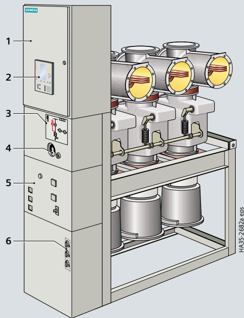
单母线开关柜 8DA10
