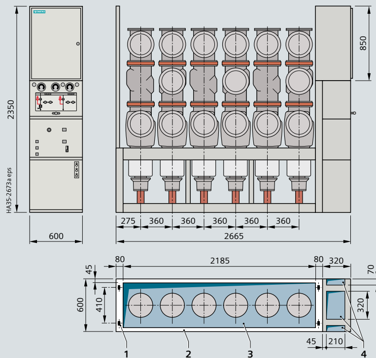
母线分段柜，带柜体联结，最大电流2500 A (母线系统1 和2)
