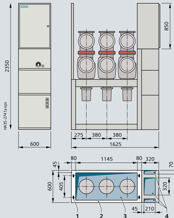
电缆连接柜, 最大电流 2500 A
