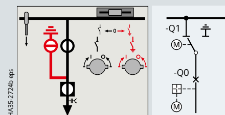
馈线合闸
