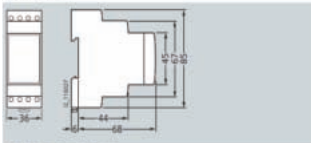
RCM 標準式, 55VB 000-6KK
