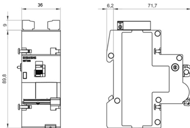
5ST3055\5ST3056\5ST3057\5ST3058
