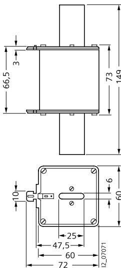
3NE1 33..-0, 3NE1 33..-2
