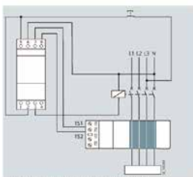
剩余电流监测装置, SSV8000-4KK, 欠电压脱扣器 (UR)
