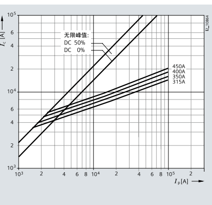
截断电流特性图 (50Hz)
