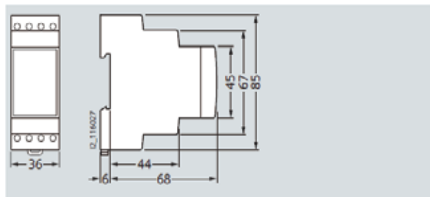
RCM 模拟式, 5SV8 000-6KK
