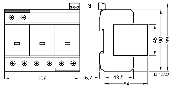
3+0 5SD7 413-1
