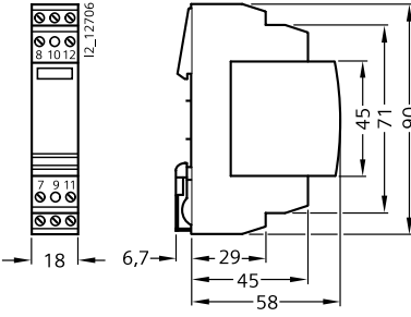
1+1 5SD7 432-
