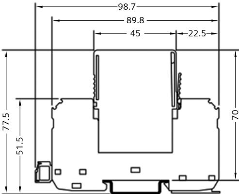
3+1 5SD7 474-3CC
