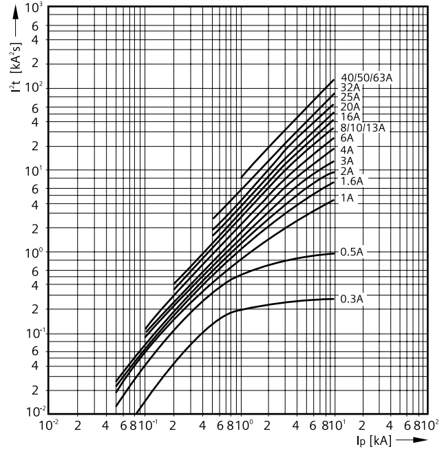
D特性
