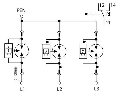
3+0 5SD7 413-1
