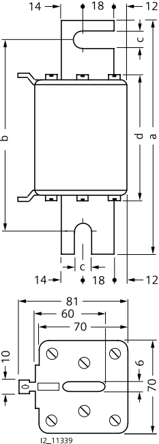
3NE3 4..
