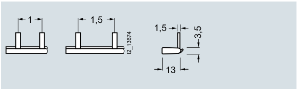
5ST3 700 5ST3 701
