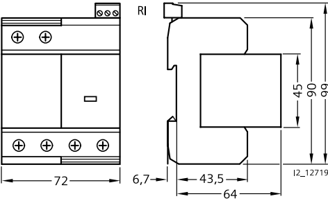
1+1 5SD7 412-1
