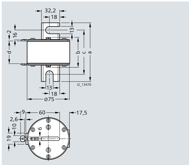
3NC3 2..-1, 3NC3 3..-1
