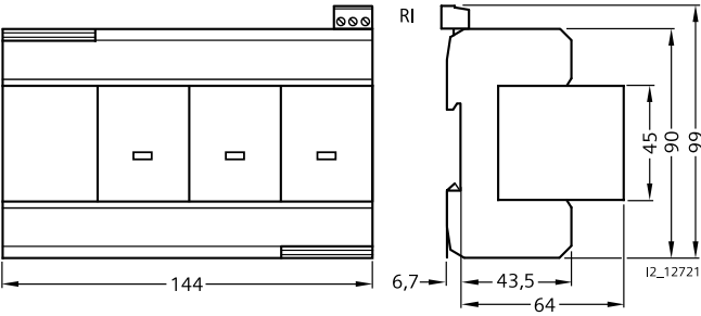
3+1 5SD7 474-3CC
