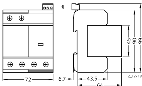
3+1 5SD7 414-1
