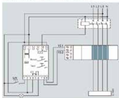
剩余电流监测装置, SSV8001-6KK, 欠电压脱扣器 (UR)
