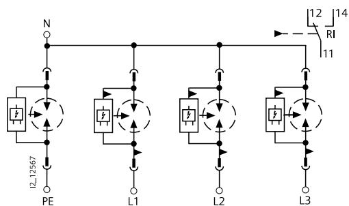
3+1 5SD7 414-1
