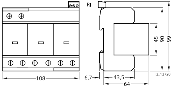
3+0 5SD7 413-1
