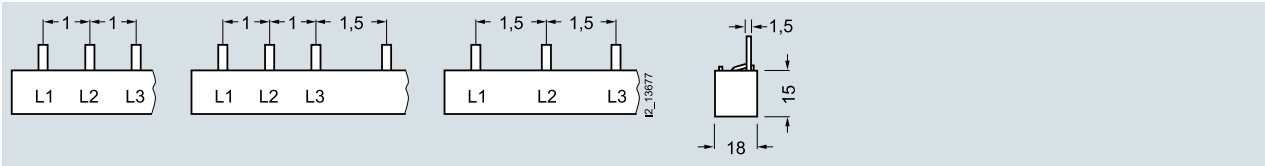
5ST3 708 5ST3 710
