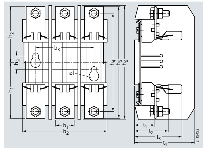
3NH4232 2C
