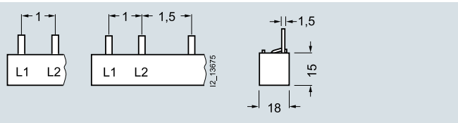
5ST3 704 5ST3 705
