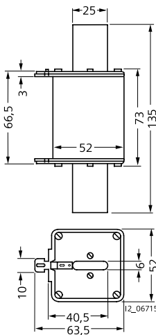
3NE1 2..-0, 3NE1 2..-2
