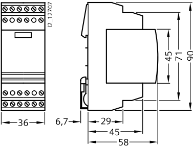
3+1 SD7 434-1
