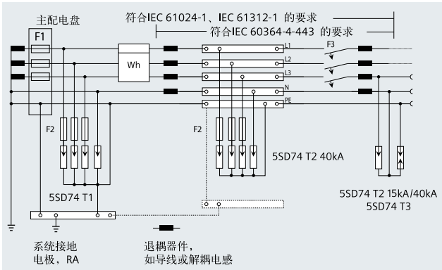
TN-S系统：可用类似TT系统的“3+1”接法
